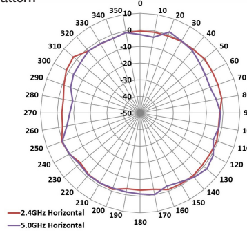
H-Plane Pattern
