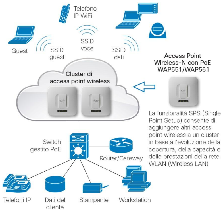
Figura 1. Configurazione tipica
